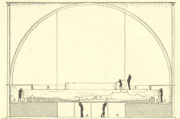
Ryc. 7. Szkic projektu Panoramy Plastiknej Dawnego Lwowa: pawilon, w nim: 2 — obraz tła, 3 — model, 4 — korytarz ruchomy, 5 — pokład górny, 6 — sala peryskopów.
